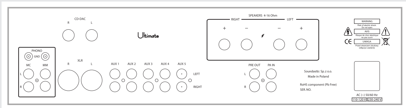
Rys. 2. Panel tylni wzmacniacza
