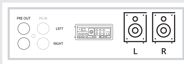
Rys. 10. Zewnętrzne wzmacniacze mocy
