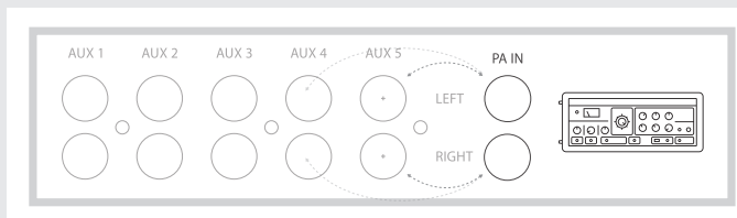
Fig. 11. Amplificateurs externes
